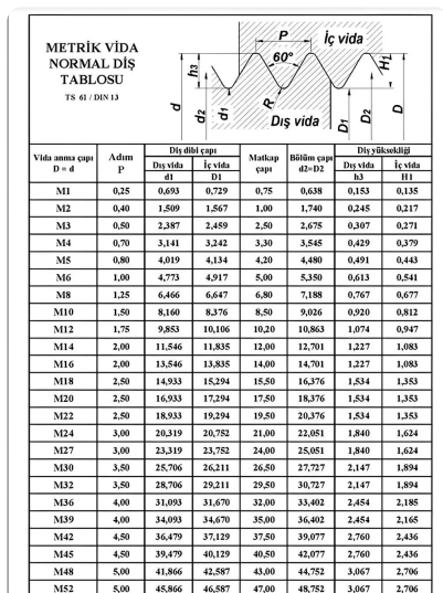
metrik diş açma toplosu
