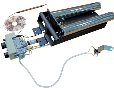
Газовая горелка с пьезорозжигом УГ-САБК-АК-12-1
