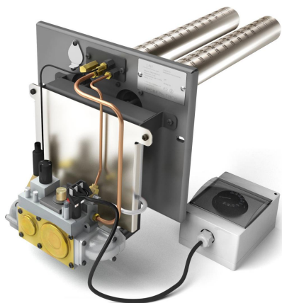
Газовая горелка ТМФ (TMF) Сахалин-1 32 (газовая горелка энер)
